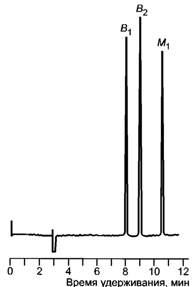
Рисунок 2 — Хроматограмма рабочего раствора смеси афлатоксинов
